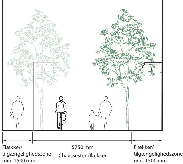
Principsnit - Storegade 1:100
